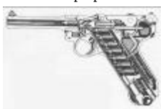
P-08. Desarrollada por Georg Luger sobre el modelo de Hugo Bochard. Tuvo problemas de alimentación. El cierre articulado es delicado. El sistema de disparo es inseguro.
