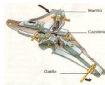
Esquema de llave de rueda. (16)
